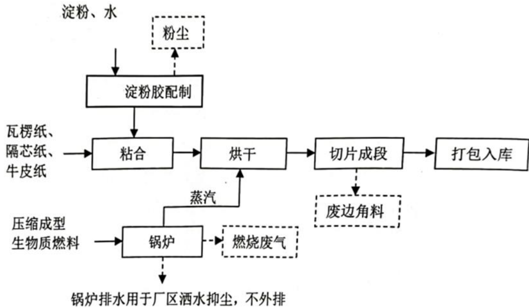
产品生产工艺流程图
